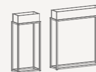
Andrea U J240 W:440 H:980 D:240 Módulo de jardinería de 400. 400 planter module.
